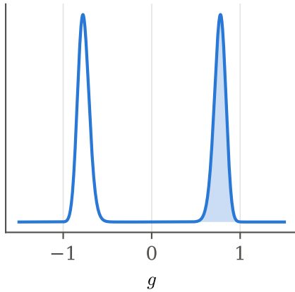
posterior p(g|d) , flat prior
