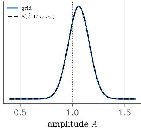
GW: template amplitude
