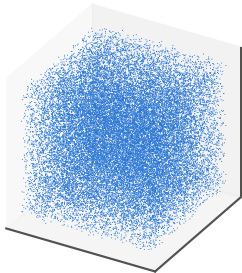
PCG64
