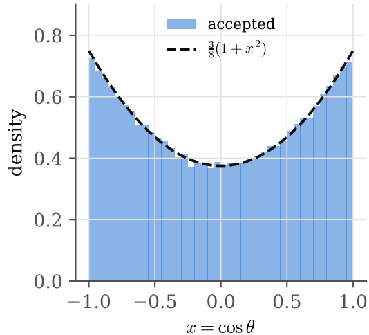
muon-pair angle
