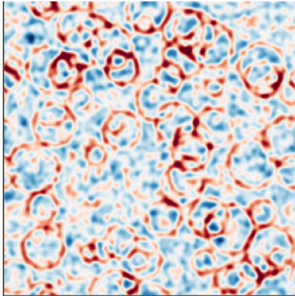
(d) |\delta_k| of blobs, phases of rings
