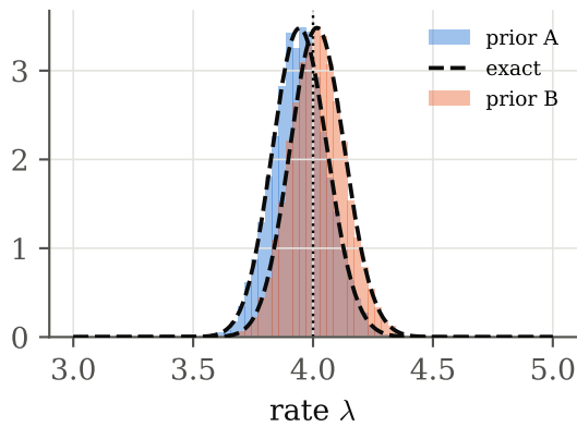
(d) posteriors, N = 300
