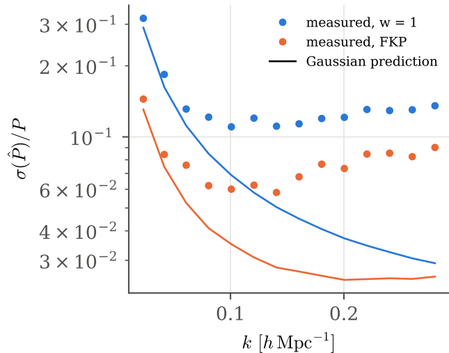
scatter
