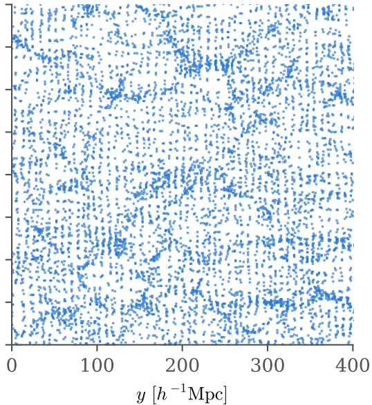
redshift space
