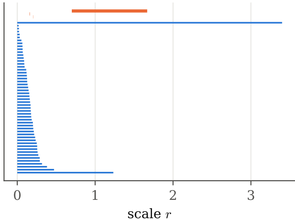
barcode ( H_0 blue, H_1 orange)
