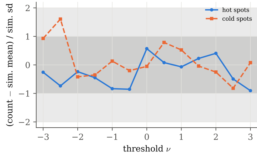
a Gaussian 'data' sky
