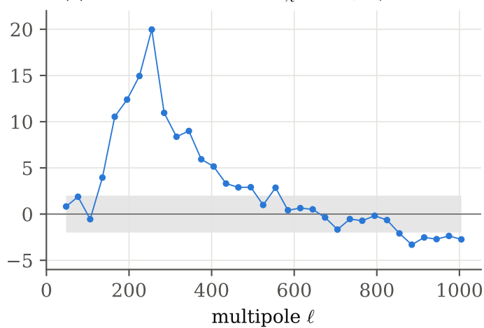
(d) half-mission difference: \chi^2 = 1312/33 , PTE 0.00
