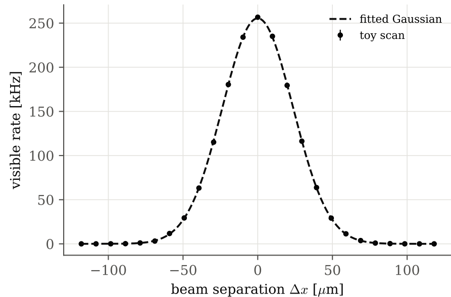
(a) a van der Meer scan
