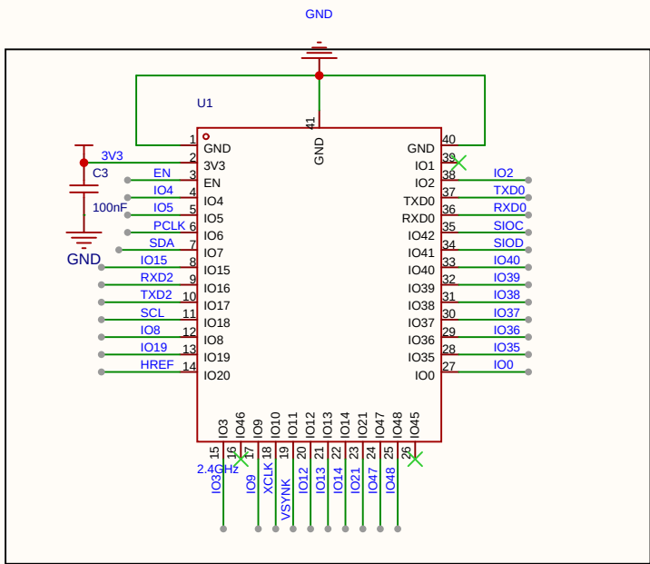
主控电路
