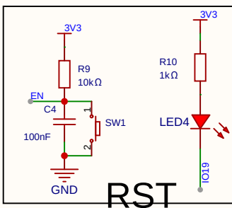
RST
