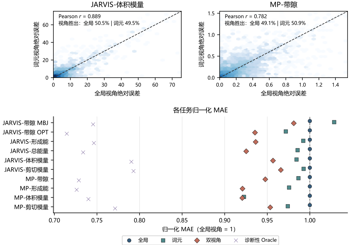
图 4: 代表性逐样本误差互补性分析。上方为两个代表任务的六边形分箱密度图, 包含 y = x 、Pearson r 和 Global/Token 路径胜出比例; 下方为十项任务中 Global、Token、固定预测级组合和诊断性 Oracle 的归一化 MAE。Oracle 使用真实标签, 不可部署; 图中展示一次代表性运行, 两次运行的定量范围见表 6。
