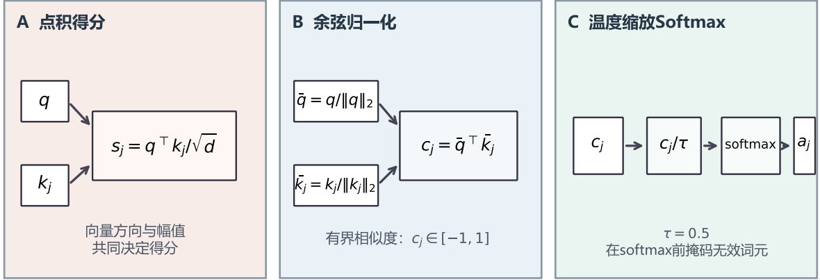
图 3: 图条件词元注意力机制。原始点积同时受向量方向与幅值影响, 余弦归一化限制相似度范围, 温度缩放 softmax 将归一化得分转化为掩码注意力权重。图中不包含实测注意力数值。
