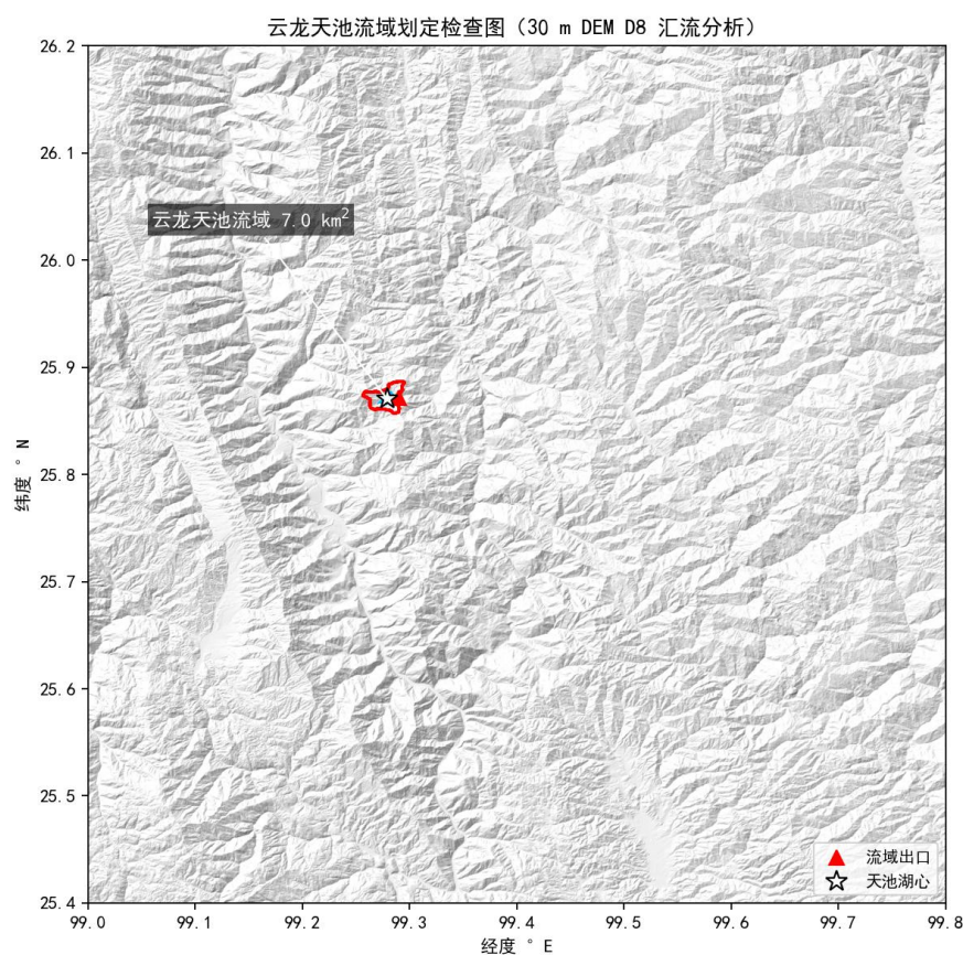
图 1 云龙天池流域位置与流域划定（基于 30 m DEM 的 D8 汇流分析；红色闭合线为流域边界，黑色五角星为湖心，红色三角形为流域出口，流域面积约 7.0 km 2 ）
