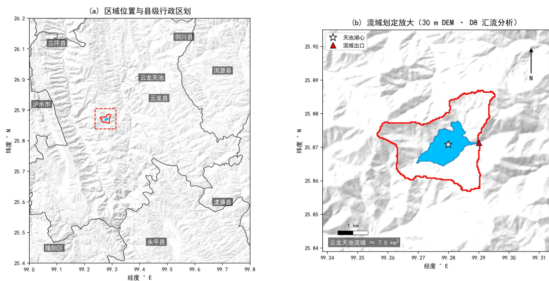
图 1 云龙天池流域位置与流域划定：(a) 区域位置与县级行政区划（底图为 GLO-30 30 m DEM 山体阴影，行政界线据阿里云 DataV 公开数据绘制，红框为(b)所示范围）；(b) 基于 30 m DEM 的 D8 汇流分析流域放大图（红色闭合线为流域边界，蓝色为天池湖面，黑色五角星为湖心，红色三角形为流域出口，流域面积约 7.0 km 2 ）
