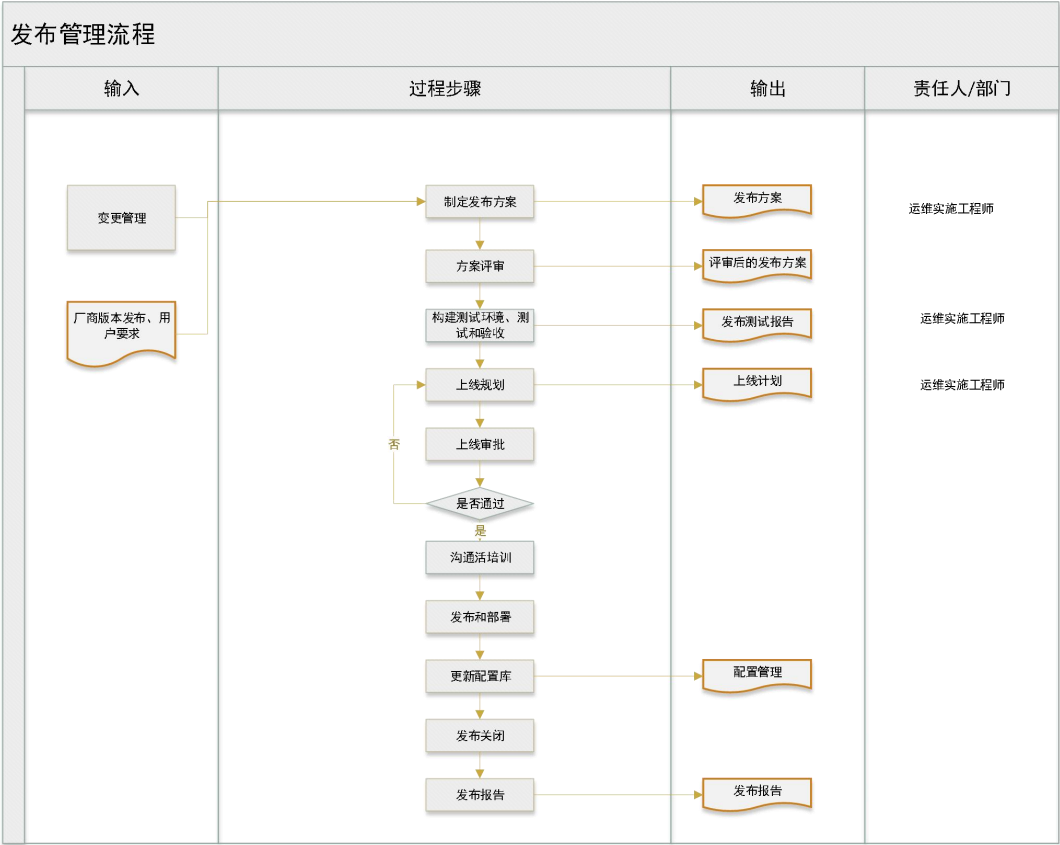
图 5-1 发布管理流程
