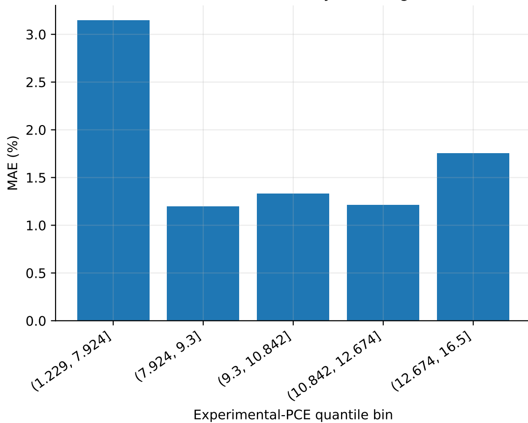
(d) Error stratified by PCE range
