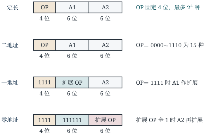
短操作码不能是长操作码的前缀，否则译码歧义（哈夫曼前缀性质）
