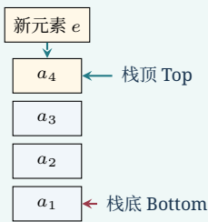
入栈: e 压到栈顶; 出栈: 弹出栈顶元素 (后进先出 LIFO)
