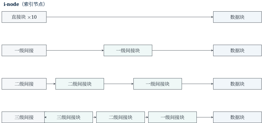
直接块数决定小文件无需间接层；文件越大，间接层越多，可支持的文件上限越大
