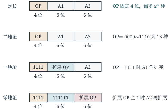
短操作码不能是长操作码的前缀，否则译码歧义（哈夫曼前缀性质）
