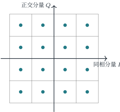
16-QAM 星座图：4 振幅 × 4 相位 = 16 个星座点，每码元携带 \log_2 16 = 4 bit
