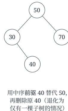
(3) 删除有两棵子树
