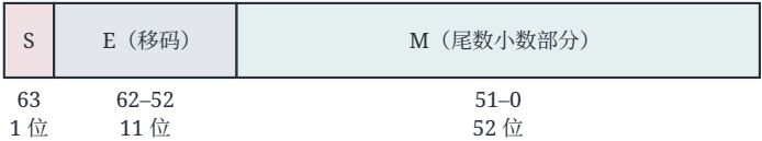
双精度 (double) 64 位
