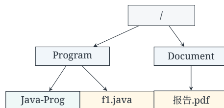
绝对路径 /Program/f1.java；相对路径（当前在 /Program）：f1.java
