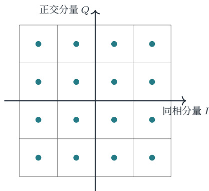
16-QAM 星座图：4 振幅 \times 4 相位 = 16 个星座点，每码元携带 \log_2 16 = 4 bit
