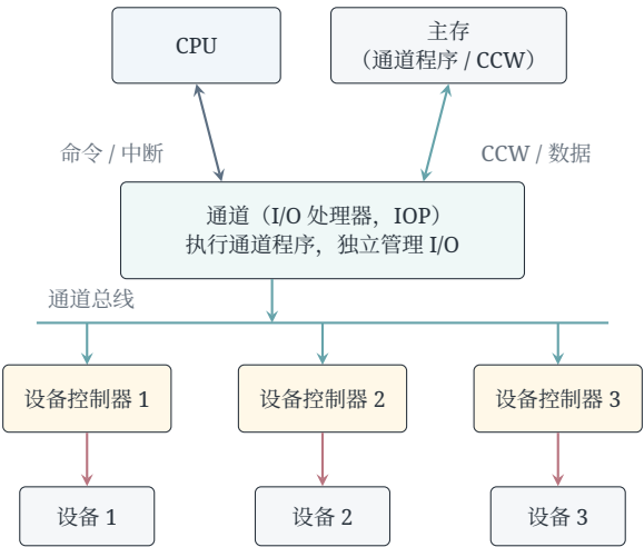
选择通道：一次只为一个高速设备服务；字节多路通道：可轮流为多个低速设备服务
