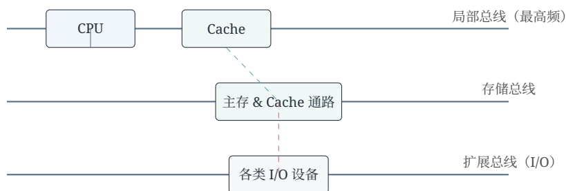
三级总线分层，速度由快到慢：局部总线 → 存储总线 → 扩展总线
