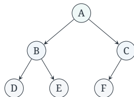
完全二叉树：最后一层从左到右连续 ( n = 6 )
