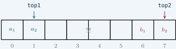
共享栈：栈 1 从低地址向高地址增长，栈 2 从高地址向低地址增长 判满条件：top1 + 1 = top2 (两栈顶指针相邻)
