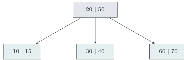
一棵 3 阶 B-树：根结点含 [20, 50]，三个孩子含 [10, 15]、[30, 40]、[60, 70] 数据结点关键字有序（如 10 < 15 ），各子树被相应关键字分隔；下层外部失败结点都在同一层
