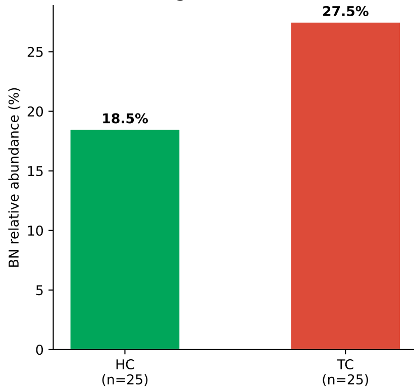
B. IgG BN (Zhang 2021, AUC=0.920)
