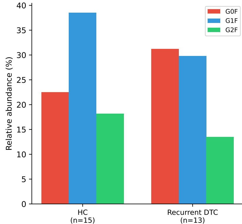
A. 糖基化 (Kudelka 2023)
