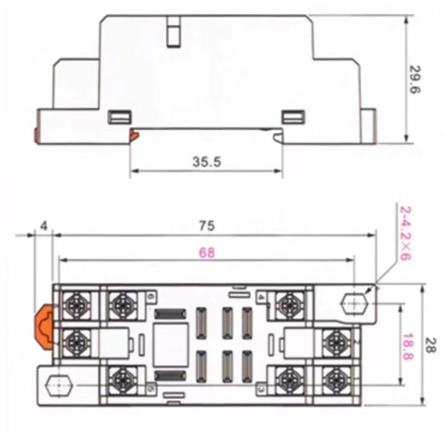
(配套底座尺寸外型)
