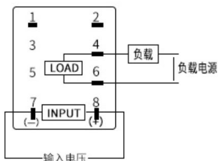
LG3-H端子配置/内部接线
