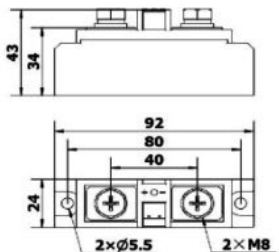
150A-200A尺寸图
