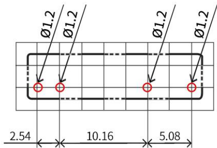
印刷电路板加工图 (BOTTOM VIEW)
