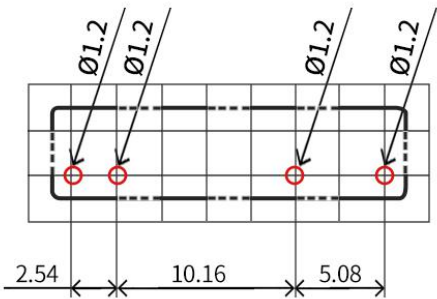
印刷电路板加工图 (BOTTOM VIEW)
