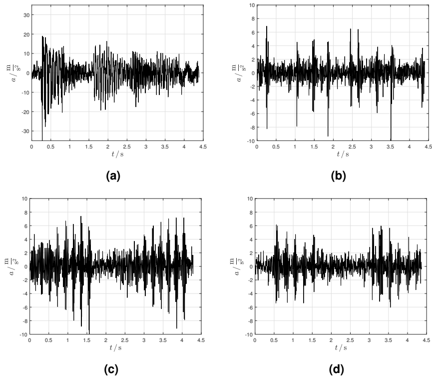
Figure 3.8 (a) Classic Mode (b) Energy Mode (c) Healing Mode (d) Recovery Mode
