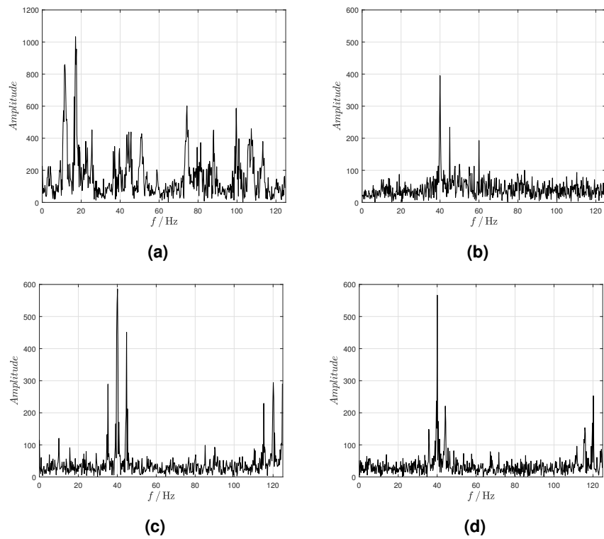
Figure 3.9 (a) Classic Mode (b) Energy Mode (c) Healing Mode (d) Recovery Mode
