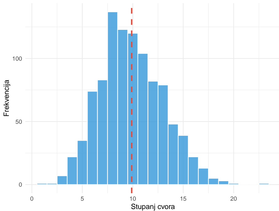
Nasumična mreža (Erdos–Renyi)
