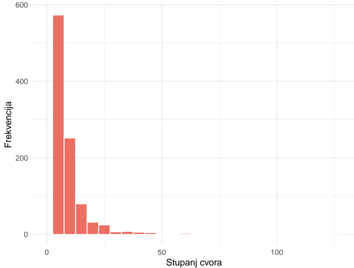
Mreža bez skale (Barabasi–Albert)
