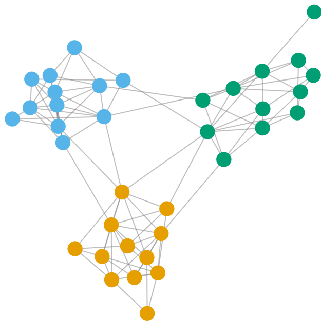
Fruchterman-Reingold
