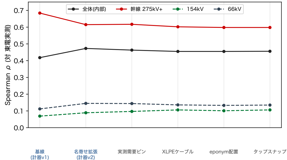
3層流れ関連の推移 — 青字=計器改訂・黒字=モデル変更（東京フルモデル）
