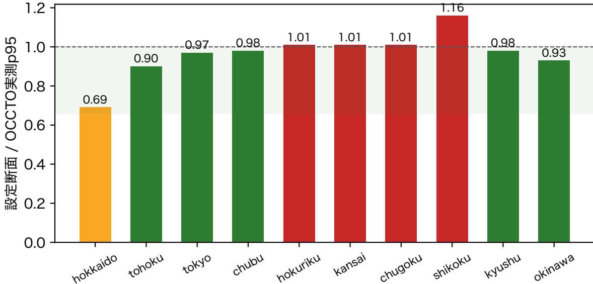
地域需要設定のOCCTO実測突合（修正前: 北海道過小・四国過大を検出→56で修正）
