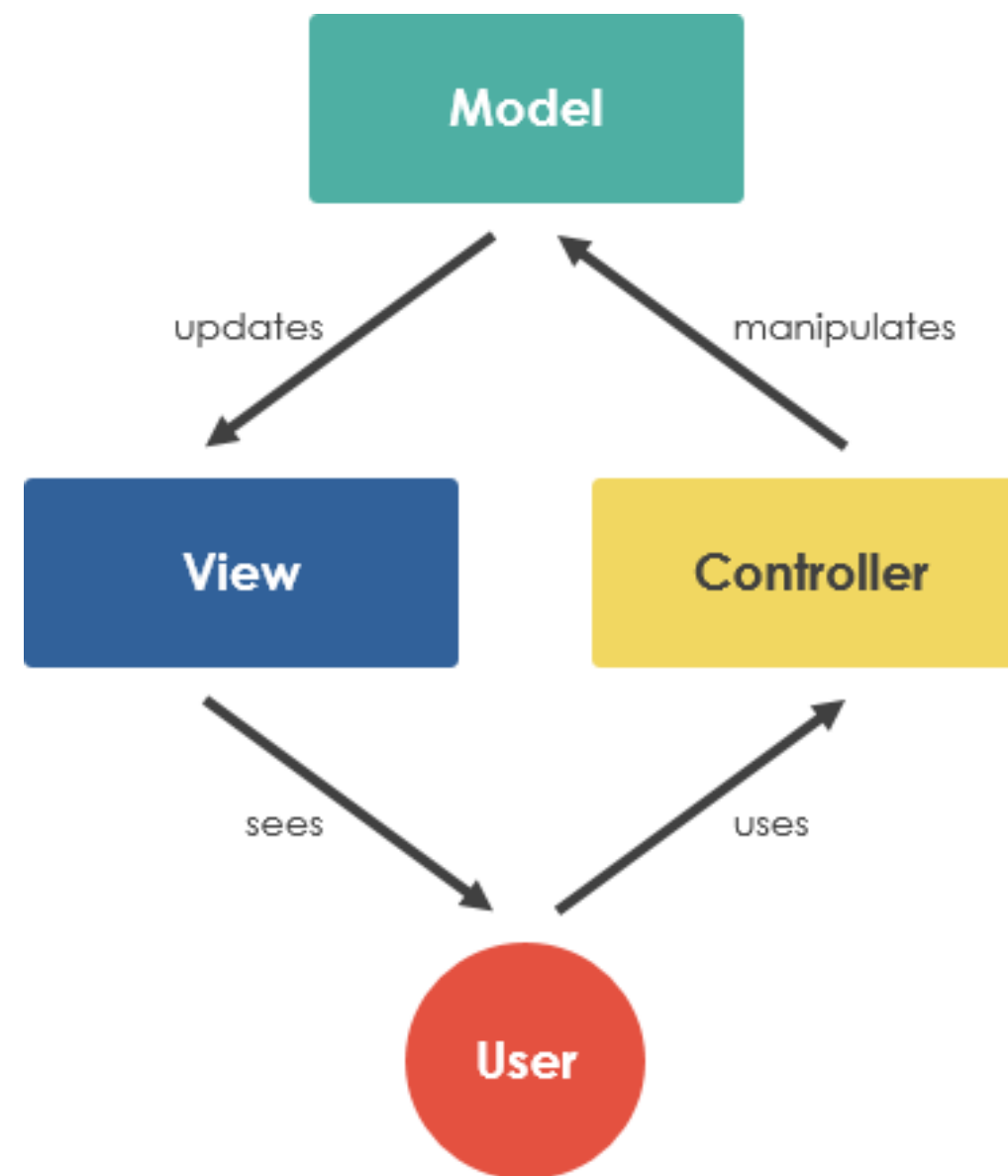
Arsitektur MVC
