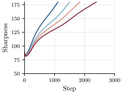
CNN
