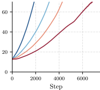
MLP
