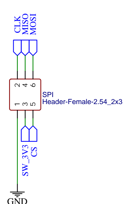
CON SPI
