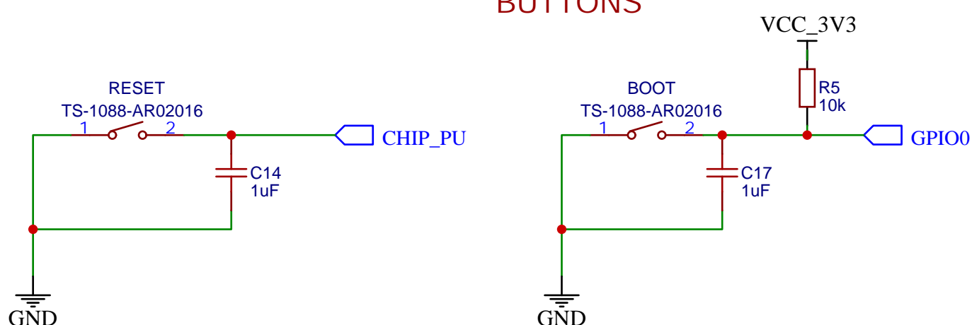
BUTTONS
