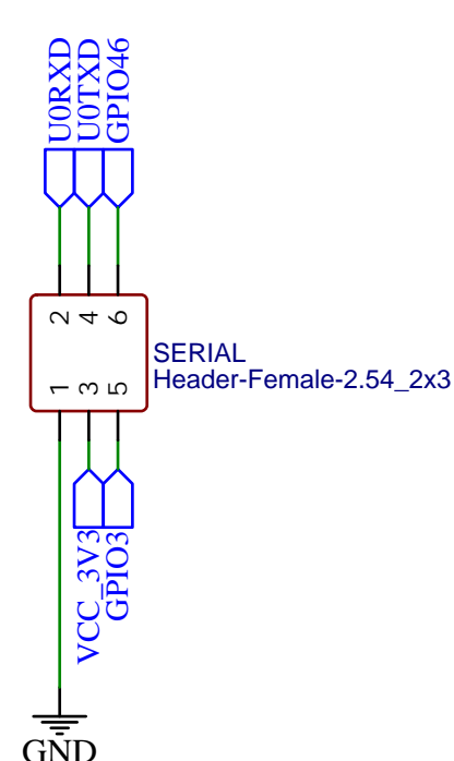
CON SERIAL
