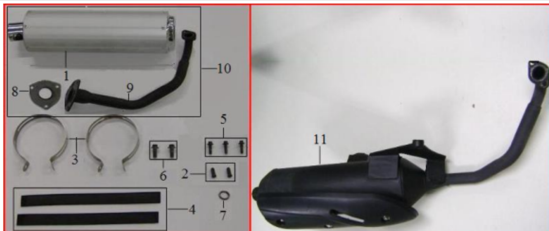
ESCAPAMENTO
