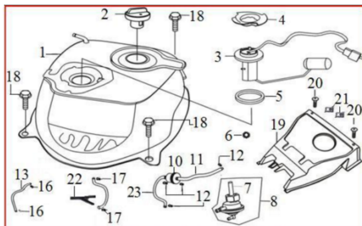
TANQUE DE COMBUSTIVEL
