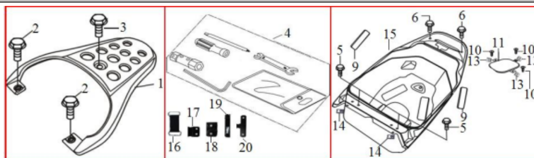
BAGAGEIRO
