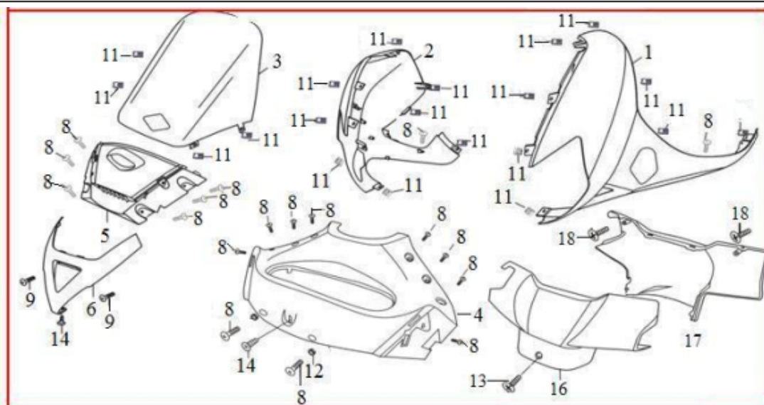
CARENAGEM FRONTAL
