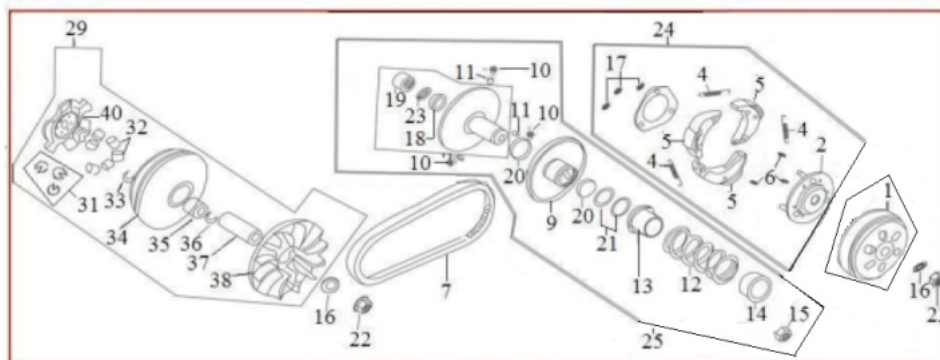
CONJUNTO DA EMBREAGEM
