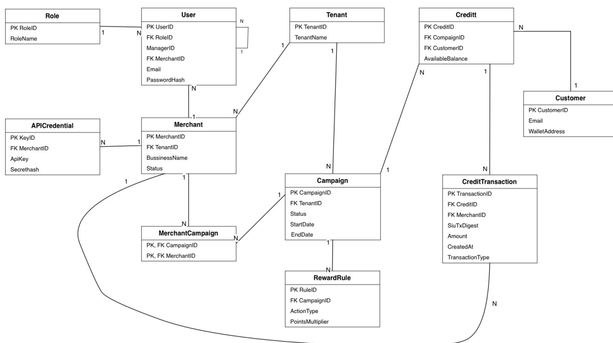
Hình 3.1: Sơ đồ thiết kế logic (Logical Diagram)
