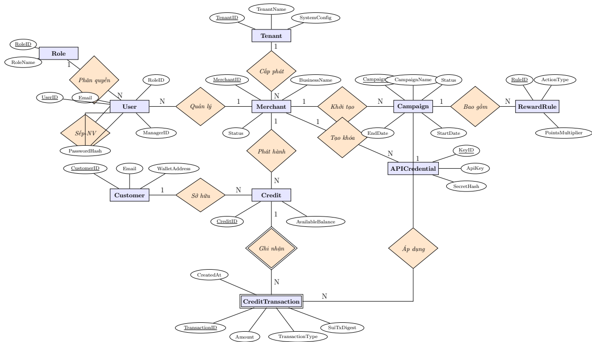
Hình 2.1: Sơ đồ Thực thể Kết hợp (ERD) mức quan niệm hệ thống OctaPoint CaaS
