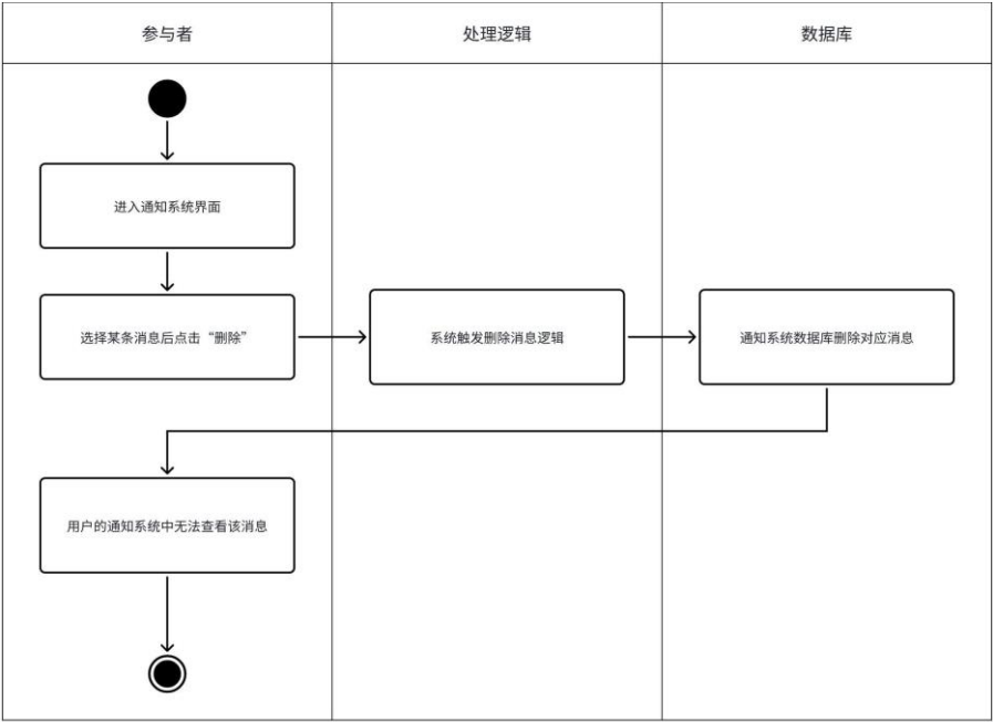
图 4.20 删除消息活动图
