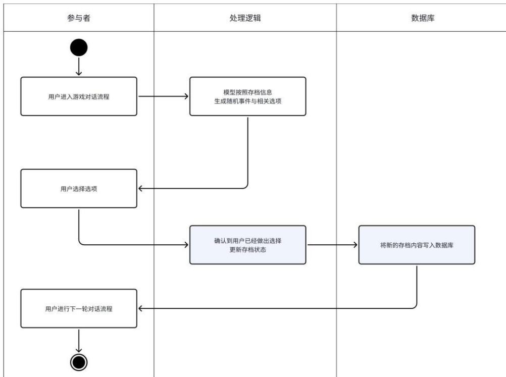
图 4.26 推进游戏活动图
