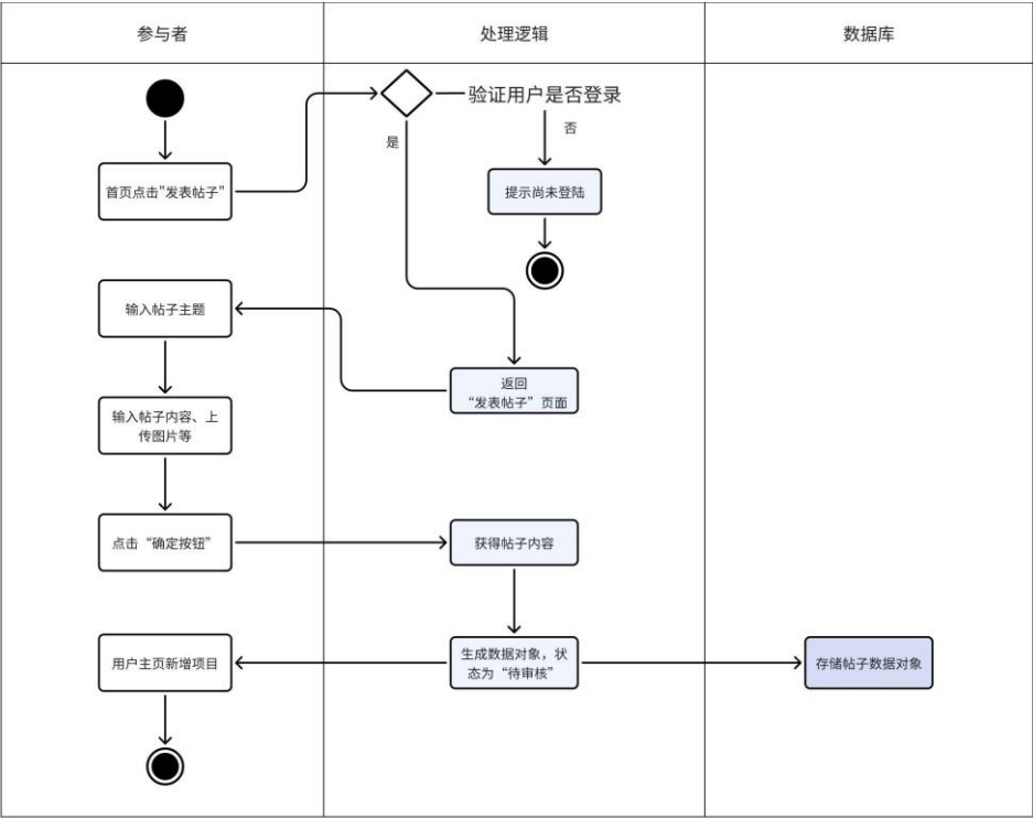
图 4.9 发表帖子活动图
