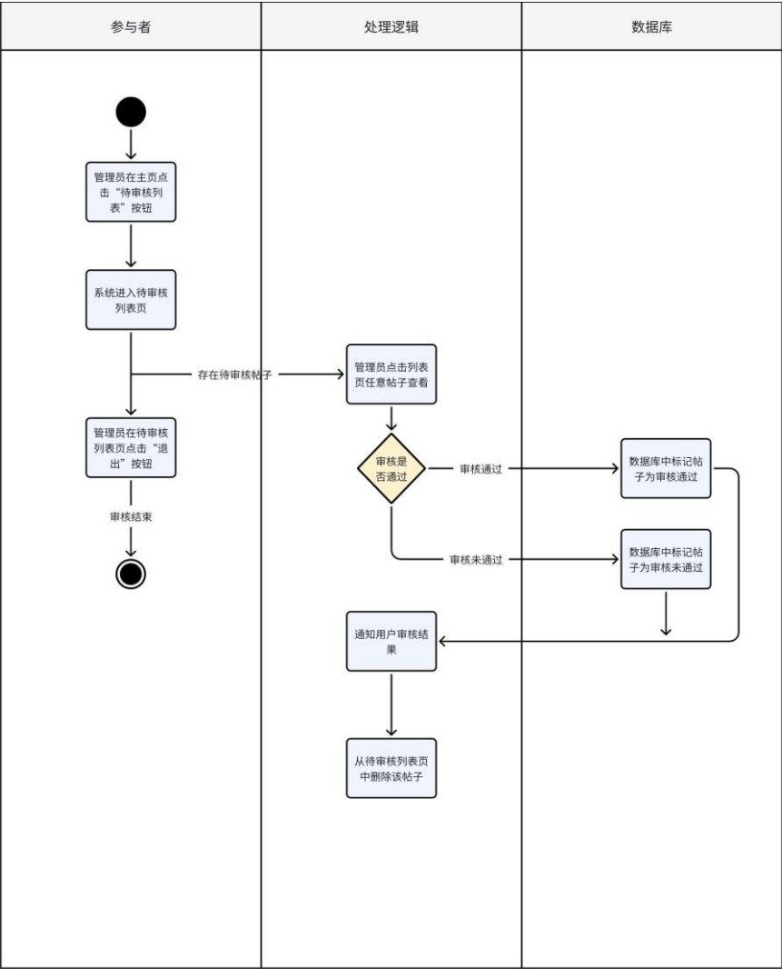
图 4.7 审核帖子活动图
