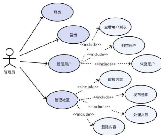
图 3.3 管理员用例图
