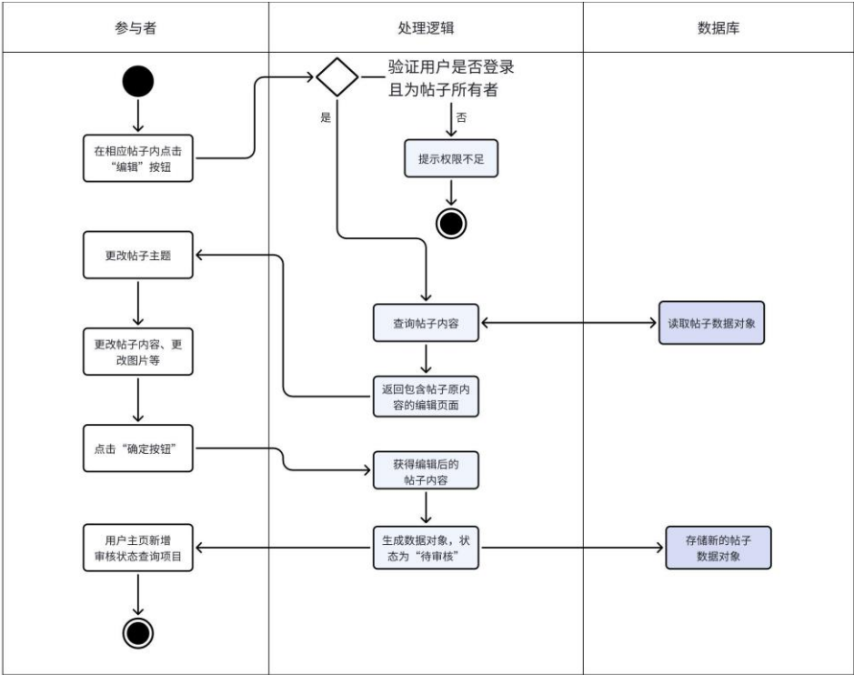
图 4.10 编辑帖子活动图
