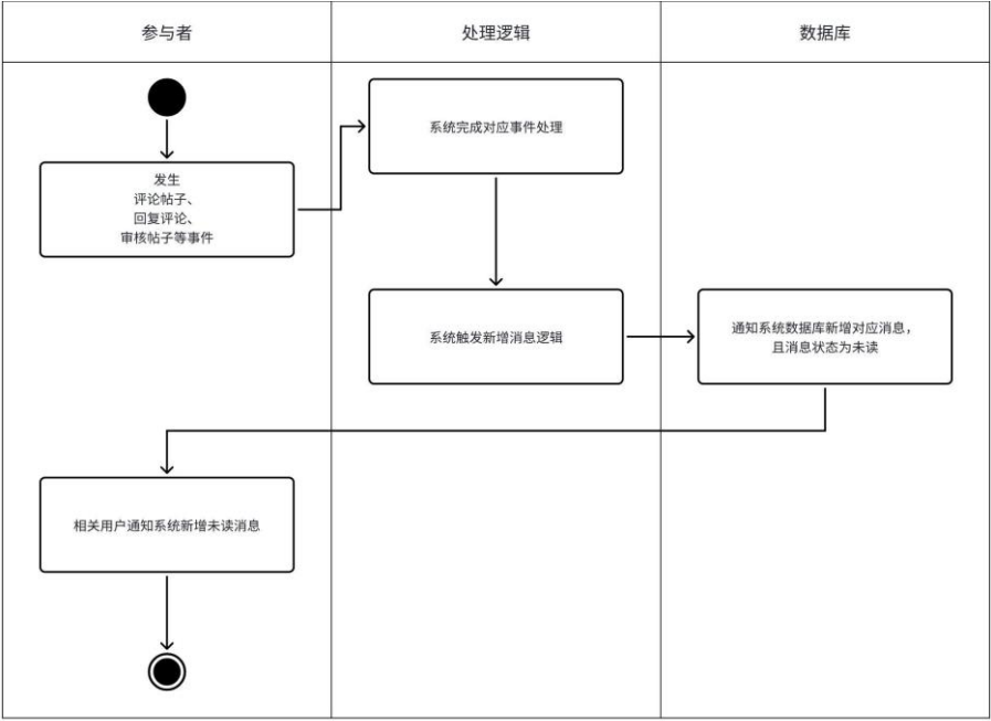
图 4.19 新增消息活动图
