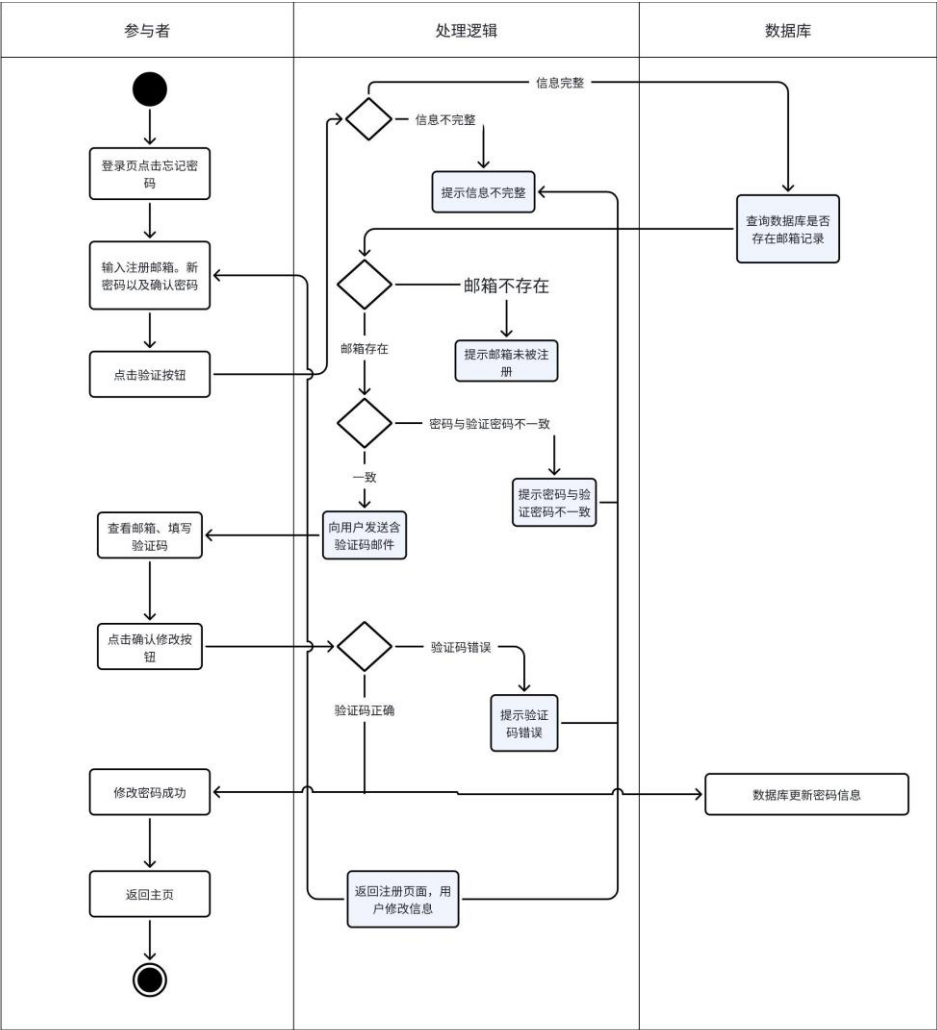
图 4.5 找回密码活动图
