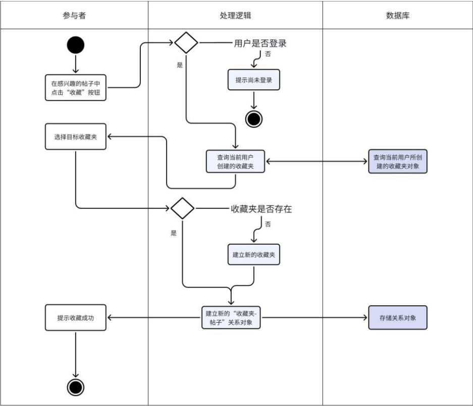
图 4.13 收藏帖子活动图
