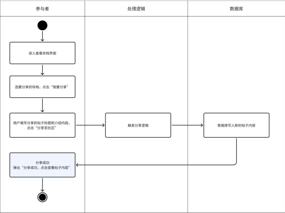
图 4.25 分享帖子活动图
