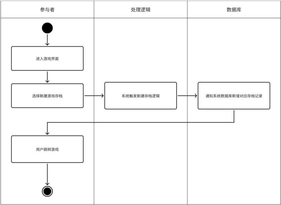
图 4.22 开始游戏活动图
