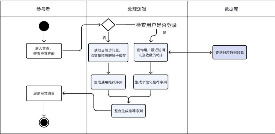
图 4.16 首页推荐活动图
