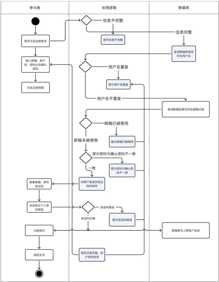
图 4.3 社区用户注册活动图
