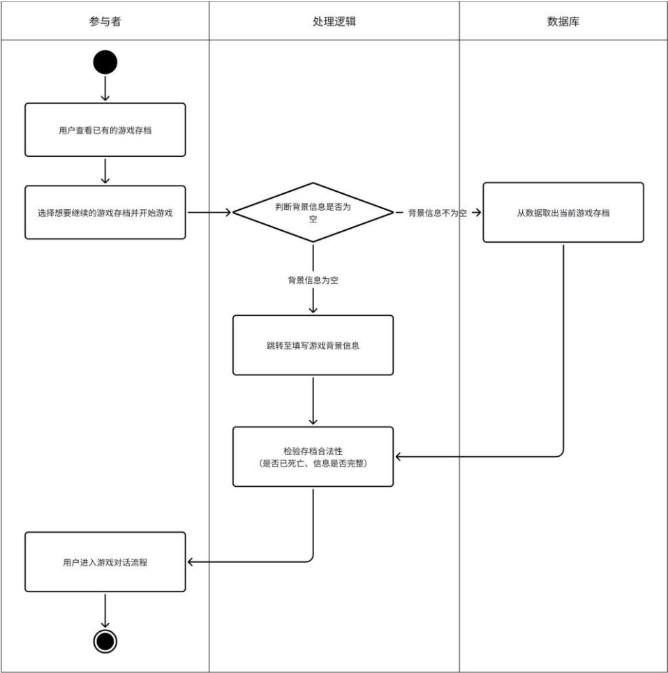
图 4.24 继续游戏活动图
