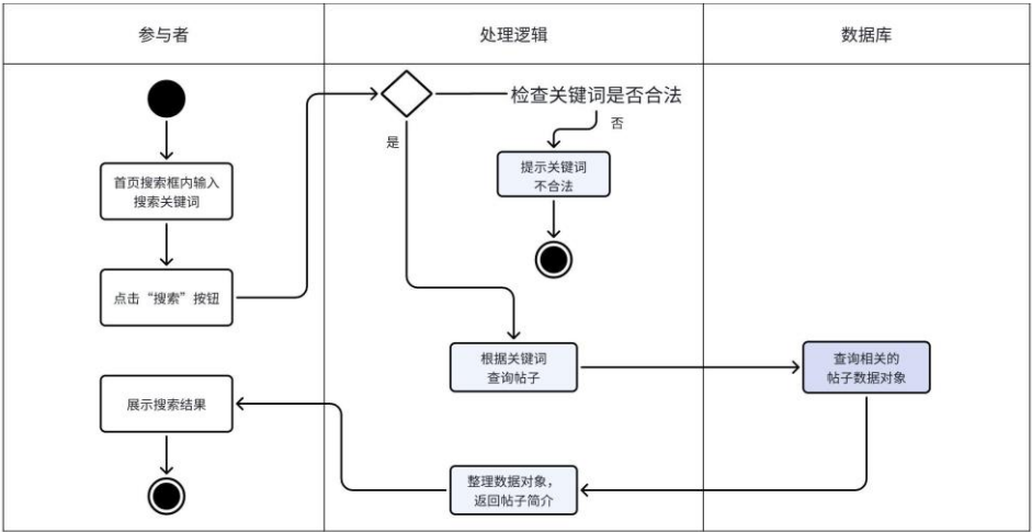
图 4.12 搜索帖子活动图
