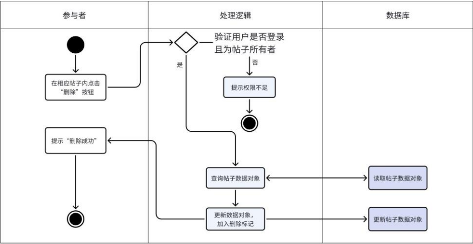
图 4.11 删除帖子活动图
