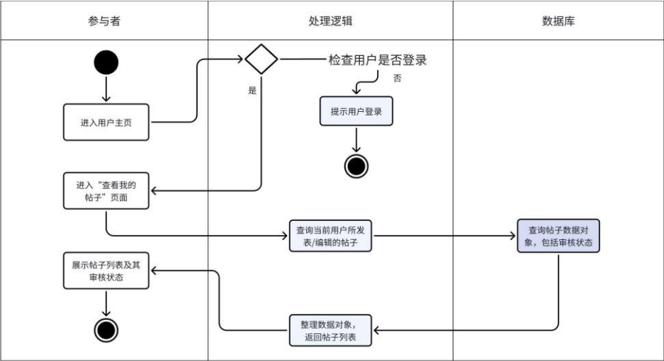
图 4.15 查询帖子审核状态活动图
