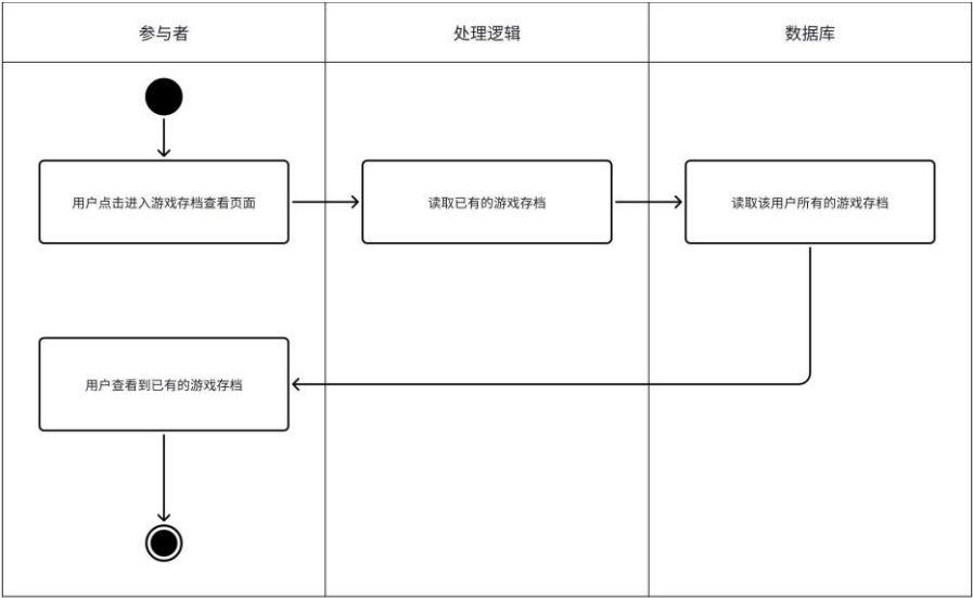
图 4.23 查看游戏存档活动图
