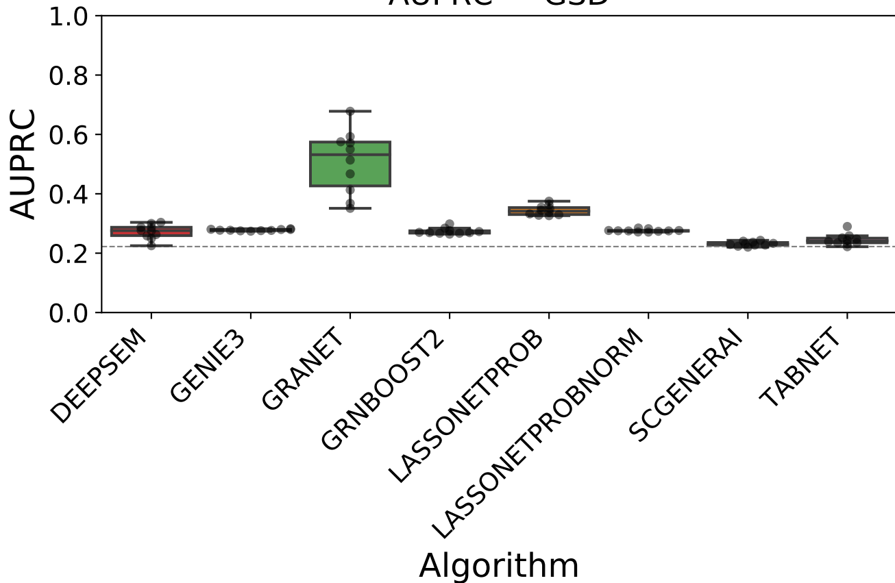
AUPRC — GSD
