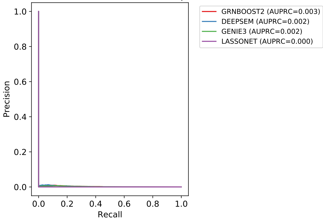
Precision-Recall — scRNA-Seq
