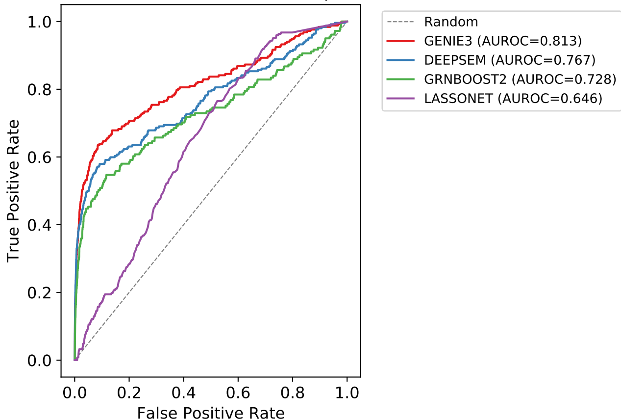
ROC Curve — scRNA-Seq
