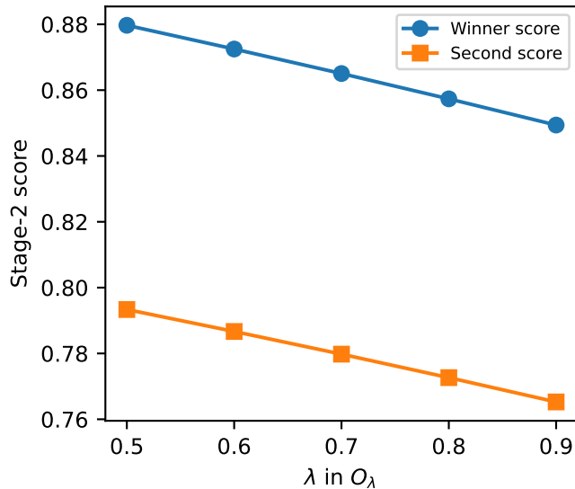
NSL-KDD
