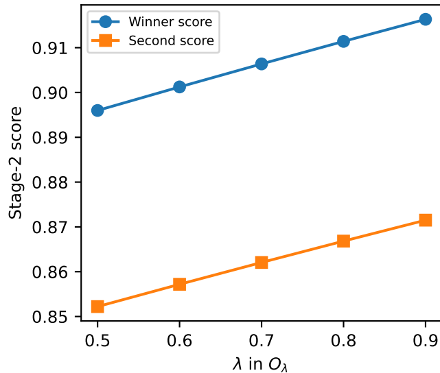
UNSW-NB15
