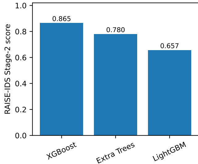
NSL-KDD
