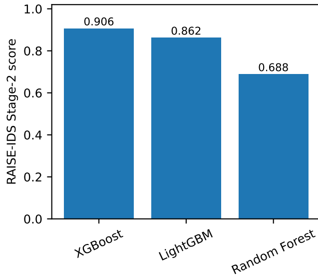
UNSW-NB15
