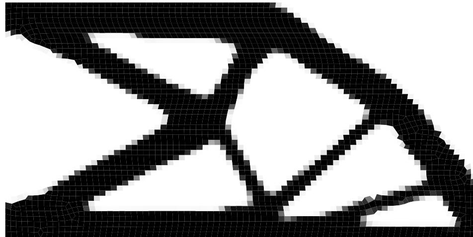
kratos optapp
