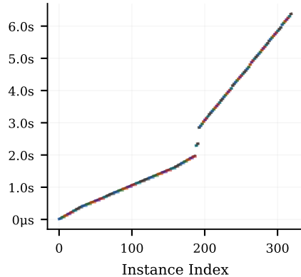
RMSNorm (LLaMA) (320 inst, 103 segs)
