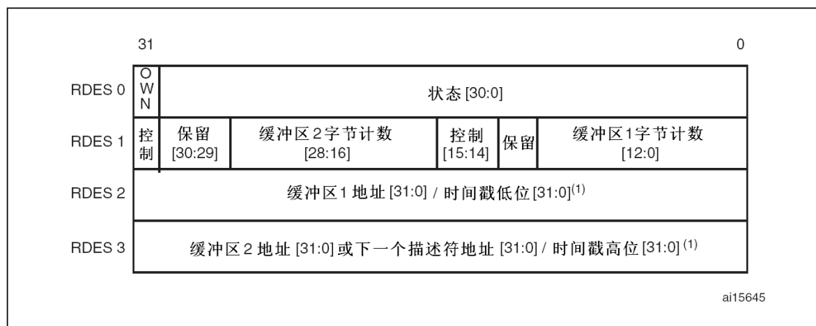
图329 IEEE1588时间戳使能时的接收描述符格式
