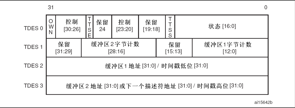
图325 传输描述符
