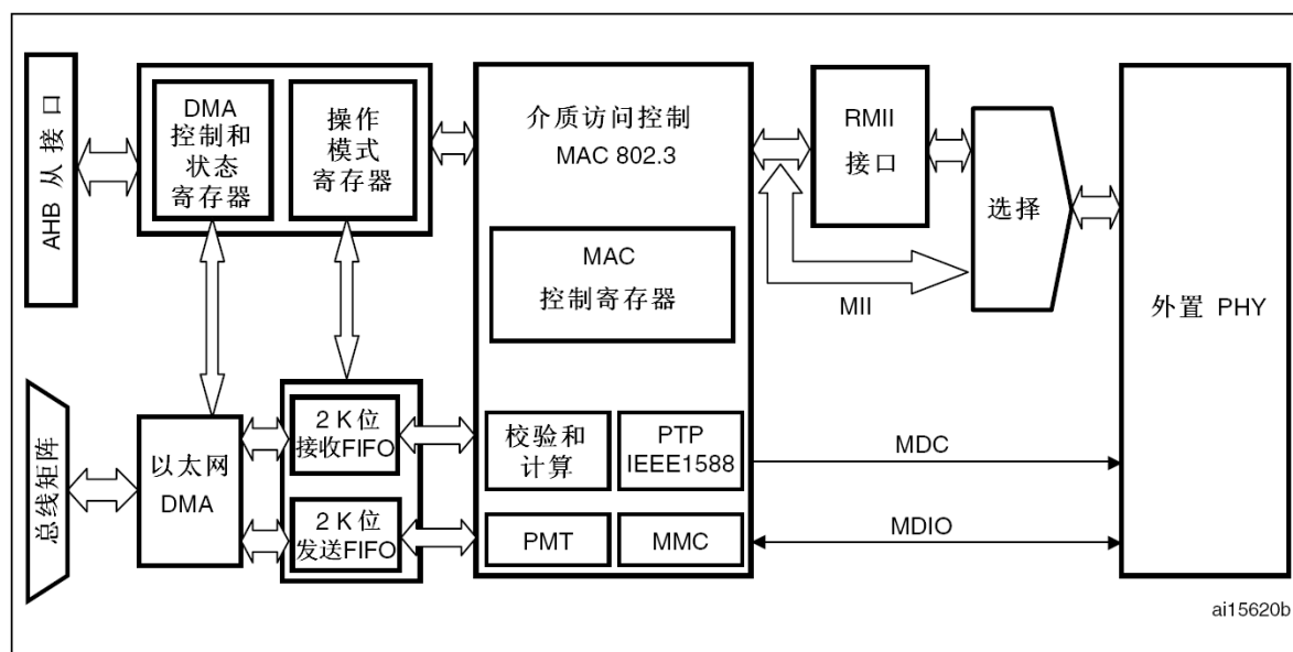
图296 ETH框图
