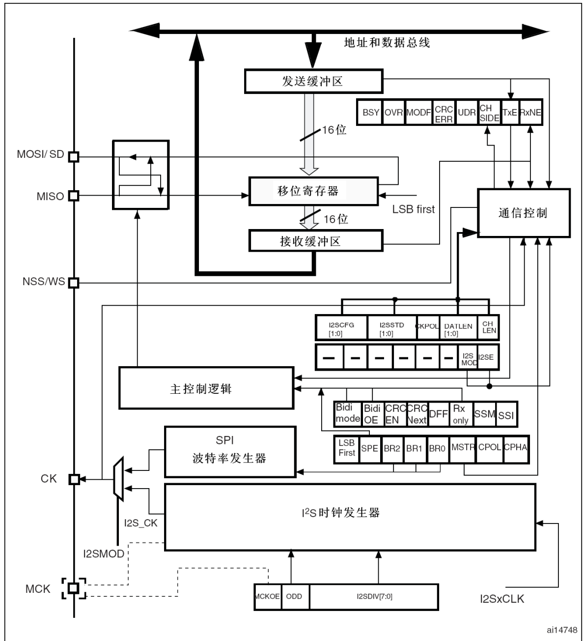
图221 I^2S 框图
