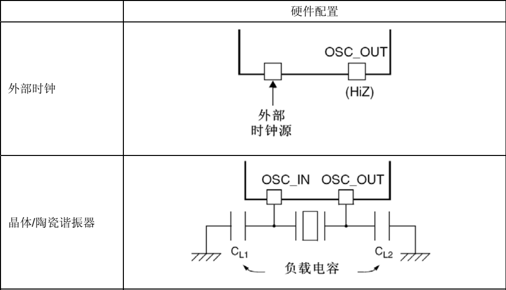
图12 HSE/LSE时钟源
